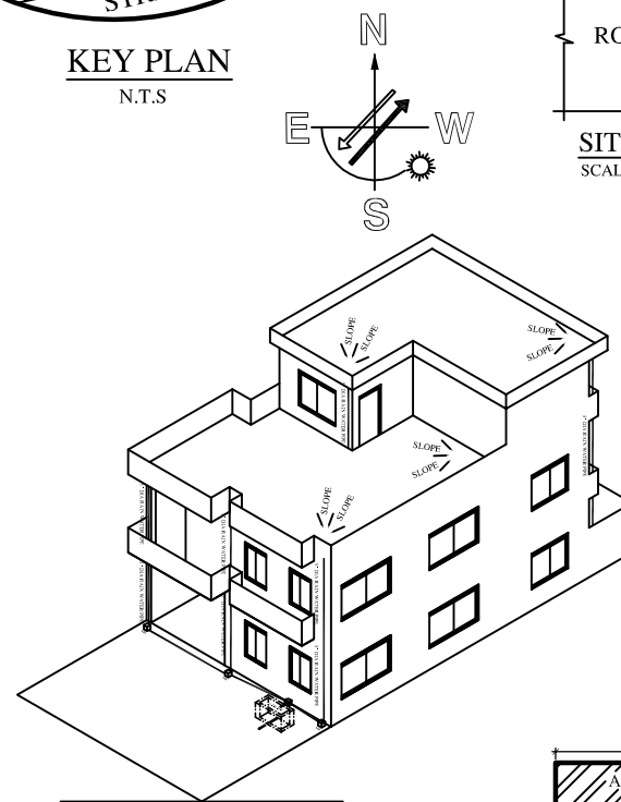
RAIN WATER SCHEME SCALE = N.T.S
