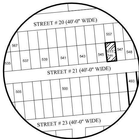
KEY PLAN Scale: NTS
